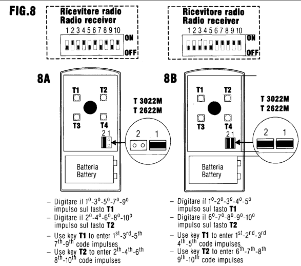
TAV. 1 - Tavola selezione canali / Channel selection table
